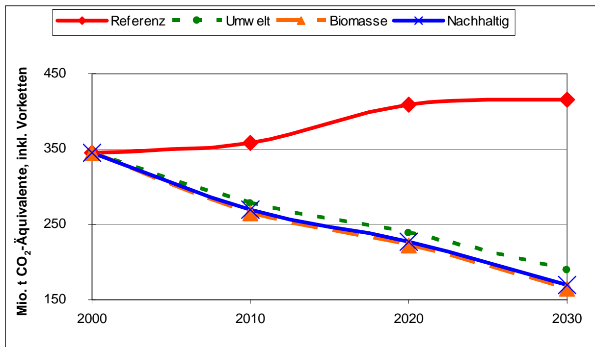
Bild 48 Treibhausgasemissionen der Strombereitstellung in den Szenarien
