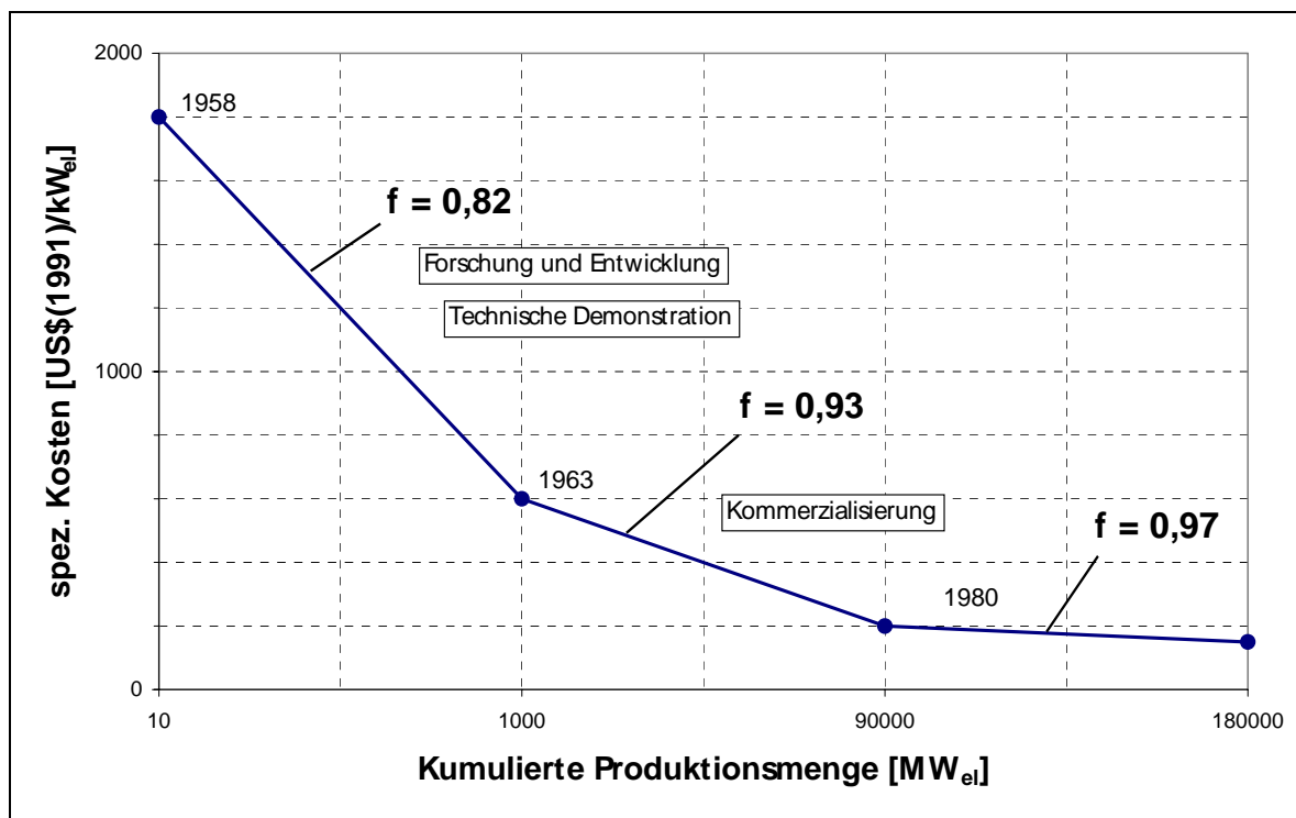
Bild 13 Präkommerzielle Kostenreduktionskurve von Gasturbinen in verschiedenen Entwicklungsphasen
